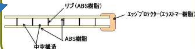
中空構造の仕組み
